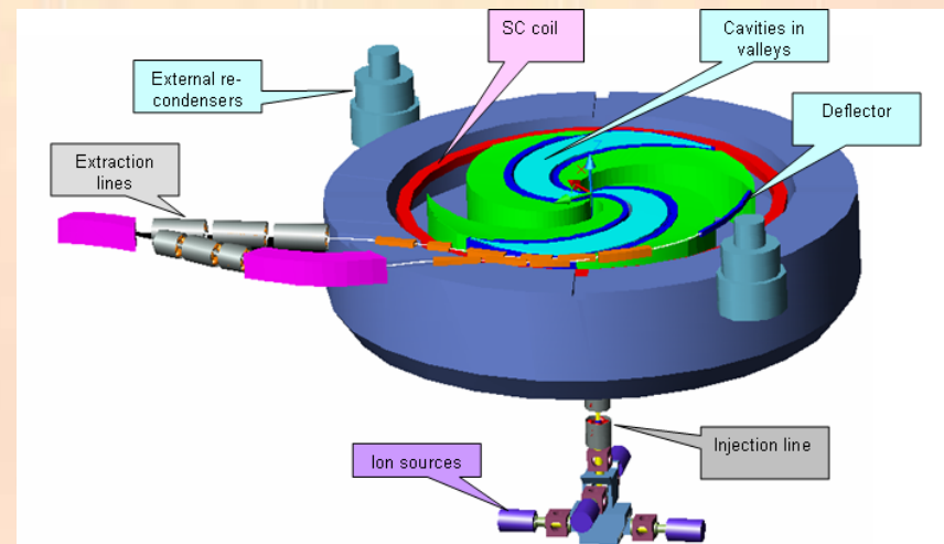
Конструктивная схема сверхпроводящего циклотрона C400 (Каен, Франция). Коллаборация IBA SA, ОИЯИ
