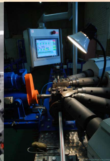
Автоматизированная экструзионная линия для производства композитных металлопластиковых труб диаметром 16...32 мм разработки и производства ООО «Экструзионные машины»
