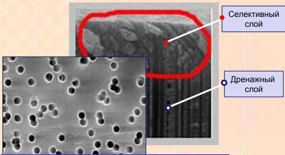
Фрагмент асимметричной трековой мембраны
