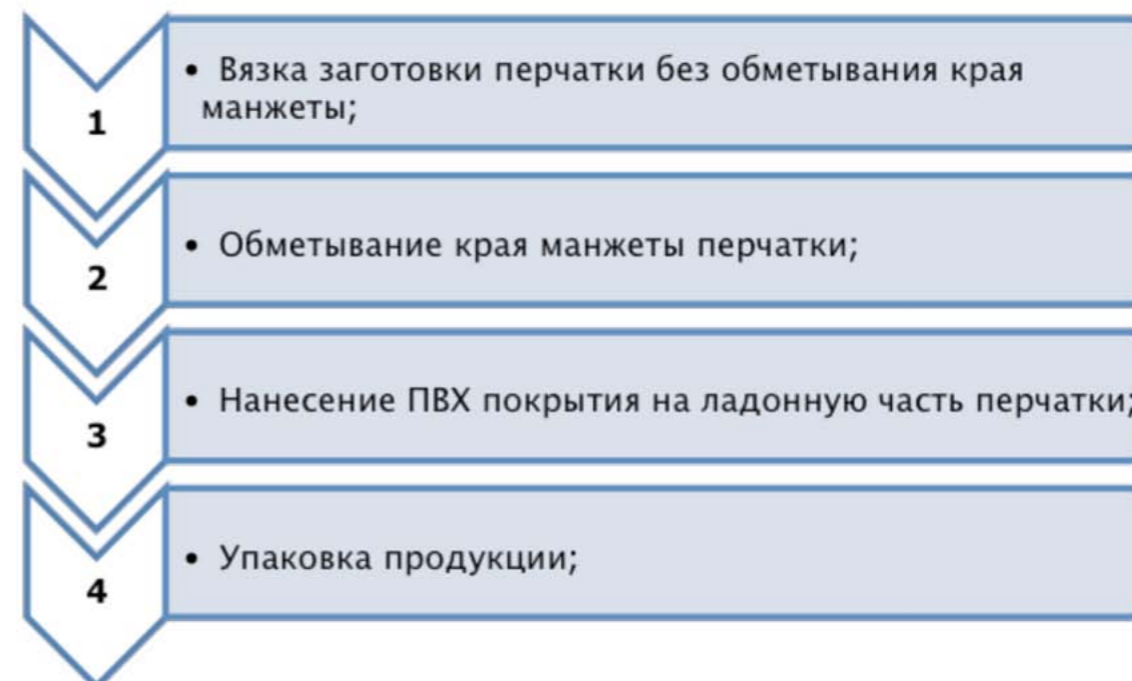
Последовательность технологических процессов производства хб перчаток
